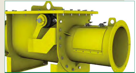
Rückschlagklappe
